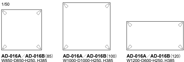
AD-016A / AD-016B (85) W850・D850・H250, H385
