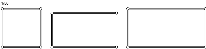
AD-006 (90) W935・D835・H700 (t 80) AD-006 (150) W1535・D835・H700 (t 80) AD-006 (180) W1835・D935・H700 (t 80)
