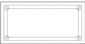
AD-002 (180) W1800・D900・ H700 (t 10) (ガラス) H710 (t 20) (突板)
