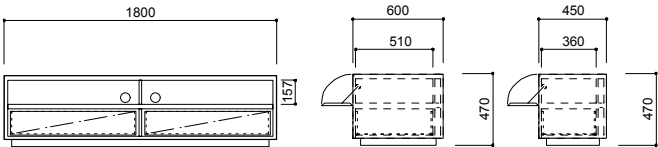
CA-017-HM W1800・D600、450・H470
