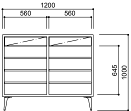
CA-012M W1200・D470・H1010 (W・H1030) (図はアルミ脚)
