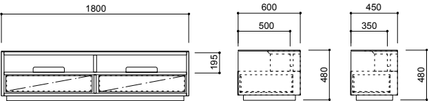
CA-017-HO W1800・D600、450・H480
