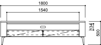
CA-016W-HC W1800・D450・H500
