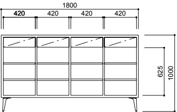
CA-012L W1800・D470・H1010 (W・H1030) (図はアルミ脚)
