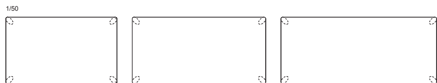
MD-905-150 W1500-D900-H720(t 50) MD-905-180 W1800-D900-H720(t 50) MD-905-210 W2100-D900-H720(t 50)
