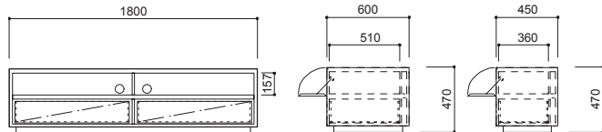
CA-017-HM W1800・D600、450・H470
