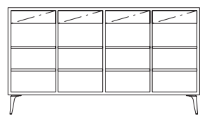
CA-012L W1800・D470・H1010 (W・H1030) (図はアルミ脚)
