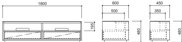
CA-017-HO W1800・D600、450・H480
