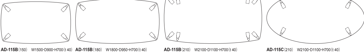
AD-115B (150) W1500・D900・H700 (t.40) AD-115B (180) W1800・D950・H700 (t.40) AD-115B (210) W2100・D1100・H700 (t.40) AD-115C (210) W2100・D1100・H700 (t.40)
