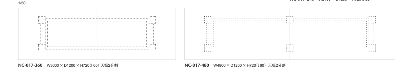
NC-017-360 W3600 × D1200 × H720 (t 60) 天板2分割
