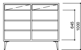
CA-012M W1200・D470・H1010 (W・H1030) (図はアルミ脚)
