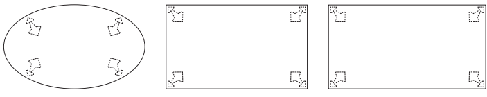
AD-892A / AD-892B(楕円形) (135) W1350・D800・H700 (t 30)
