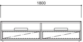
CA-017-HO W1800・D600、450・H480
