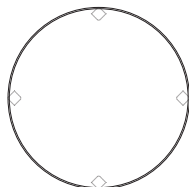
AD-083 (120C) φ1200・H700 (t 65)
