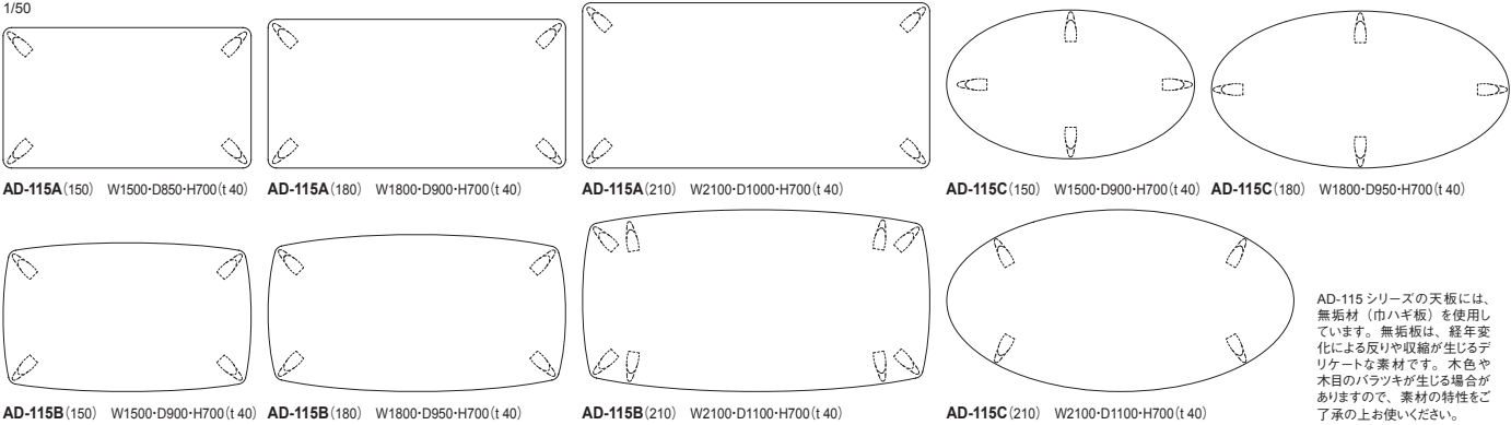
AD-115B (150) W1500・D900・H700 (t.40) AD-115B (180) W1800・D950・H700 (t.40) AD-115B (210) W2100・D1100・H700 (t.40) AD-115C (210) W2100・D1100・H700 (t.40)
