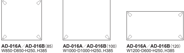
AD-016A／AD-016B (85) W850・D850・H250, H385
