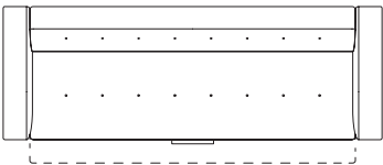
AD-235S (ソファベッド) W2270・D840 (S80)・H750 (SH400)・AH700
