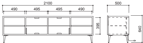
CA-002 Type-B W2100・D500・H640 (W・H660) (図はアルミ脚)
