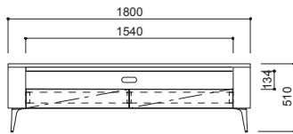
CA-016W-HC W1800・D450・H510 (W・H530) (図はアルミ脚)
