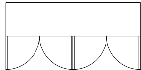
CA-012L W1800・D470・H1010 (W・H1030) (図はアルミ脚)
