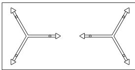
AD-062B(180) W1800-D900-H700
