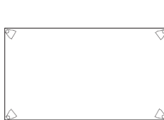
AD-004(150) W1500-D850-H700(t 30)
