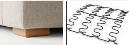
▲NC-045 木製レッグ NC-045ソファの脚部には、木製 脚を取り付けてあります。 ▲ウェーブスプリング ウェーブスプリングが座フレーム内に 使用されており、ホールド感のある座 り心地が得られます。
