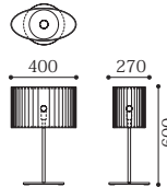
RA-031L (デスクスタンド) W400-D270-H600
