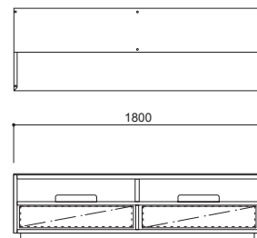
CA-017-HO W1800・D600、450・H480
