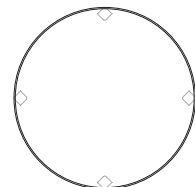
AD-083 (120C) φ1200・H700 (t 65)
