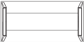
MD-1102-180 W1800・D900・ ガラス天板 H703 (t15) セラミック天板・木天板 H720 (t35)
