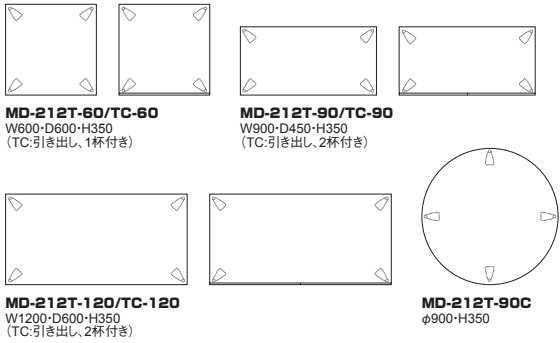
MD-212T-60/TC-60 W600・D600・H350 (TC:引き出し、1杯付き) MD-212T-90/TC-90 W900・D450・H350 (TC:引き出し、2杯付き) MD-212T-120/TC-120 W1200・D600・H350 (TC:引き出し、2杯付き) MD-212T-90C φ900・H350
