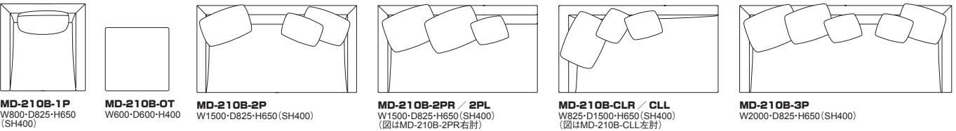
MD-210B-1P W800・D825・H650 (SH400) MD-210B-OT W600・D600・H400 MD-210B-2P W1500・D825・H650 (SH400) MD-210B-2PR / 2PL W1500・D825・H650 (SH400) (図はMD-210B-2PR右肘) MD-210B-CLR / CLL W825・D1500・H650 (SH400) (図はMD-210B-CLL左肘) MD-210B-3P W2000・D825・H650 (SH400)
