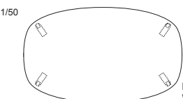
MD-502-150 W1500・D900・H700(t 45)
