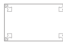
AD-892A / AD-892B (135T) W1350・D800・H700(t 30)
