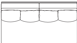
AD-085A-2P W1700・D930・H750・SH400
