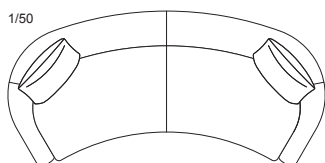
MD-3211-3PL W2100・D1035・H790 (SH400) (クッション×2)
