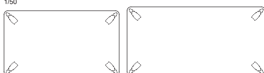
AD-115A (150) W1500・D850・H700 (t 40) AD-115A (180) W1800・D900・H700 (t 40)
