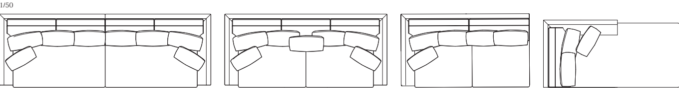
NC-009-4P (2PR+2PL) W2800 (W1400 + W1400) × D980 × H800 (SH400) AH650 (Lクッション×6 Sクッション×2) NC-009-3P W2150 × D980 × H800 (SH400) AH650 (Lクッション×5 Sクッション×2) NC-009-2LR / 2LL W1700 × D980 × H800 (SH400) AH650 (Lクッション×4 Sクッション×1) NC-009-CLL / CLR W900 × D1800 × H800 (SH400) AH650 (Lクッション×2 Sクッション×1)
