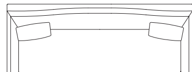
NC-046BC/C-3PL W2400 × D900 × H850 (SH400) AH650 (Lクッション×2)
