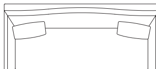
NC-046BC/C-3P W2100 × D900 × H850 (SH400) AH650 (Lクッション×2)
