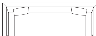
NC-055C-3PL W2400 × D850 × H720 (SH400) (Lクッション×2)
