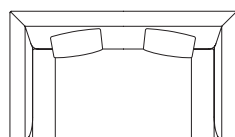
NC-055C-2P W1500 × D850 × H720 (SH400) (Sクッション×2)
