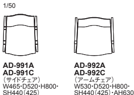
AD-991A AD-991C (サイドチェア) W465・D520・H800・SH440 (425) AD-992A AD-992C (アームチェア) W530・D520・H800・SH440 (425)・AH630
