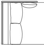
AD-085LR-LL W930・D1730・H750・SH400
