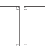
AD-025 (180) W1800・D900・H720 (t 50)
