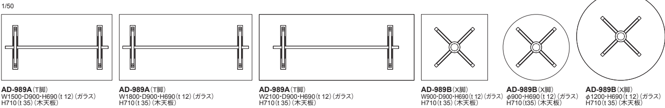
AD-989A (T脚) W1500・D900・H690 (t 12) (ガラス) H710 (t 35) (木天板) AD-989A (T脚) W1800・D900・H690 (t 12) (ガラス) H710 (t 35) (木天板) AD-989A (T脚) W2100・D900・H690 (t 12) (ガラス) H710 (t 35) (木天板) AD-989B (X脚) W900・D900・H690 (t 12) (ガラス) H710 (t 35) (木天板) AD-989B (X脚) φ900・H690 (t 12) (ガラス) H710 (t 35) (木天板) AD-989B (X脚) φ1200・H690 (t 12) (ガラス) H710 (t 35) (木天板)
