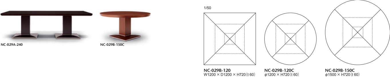
NC-029B-120 W1200 × D1200 × H720 (t 60)
