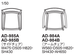
AD-985A AD-985B (サイドチェア) W475・D505・H820・SH430 AD-984A AD-984B (アームチェア) W560・D505・H820・SH430・AH650
