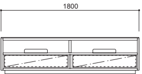
CA-017-HO W1800・D600、450・H480
