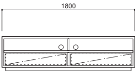
CA-017-HM W1800・D600、450・H470
