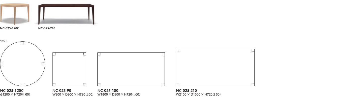
NC-025-120C φ1200 × H720 (t 60)
