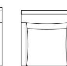
MD-506L W700・D755・H800(SH400)AH600
