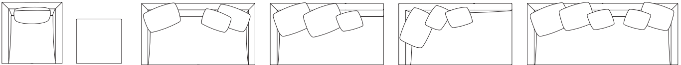
MD-210B-1P W800・D825・H650 (SH400) MD-210B-OT W600・D600・H400 MD-210B-2P W1500・D825・H650 (SH400) MD-210B-2PR / 2PL W1500・D825・H650 (SH400) (図はMD-210B-2PR右肘) MD-210B-CLR / CLL W825・D1500・H650 (SH400) (図はMD-210B-CLL左肘) MD-210B-3P W2000・D825・H650 (SH400)
