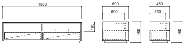
CA-017-HO W1800・D600、450・H480
