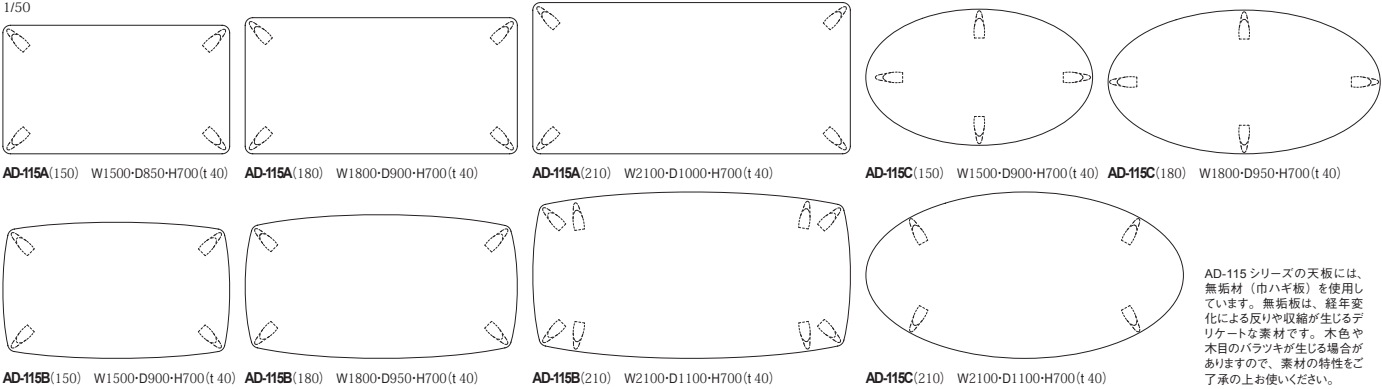
AD-115A(150) W1500・D850・H700(t 40) AD-115A(180) W1800・D900・H700(t 40) AD-115A(210) W2100・D1000・H700(t 40) AD-115C(150) W1500・D900・H700(t 40) AD-115C(180) W1800・D950・H700(t 40) AD-115B(150) W1500・D900・H700(t 40) AD-115B(180) W1800・D950・H700(t 40) AD-115B(210) W2100・D1100・H700(t 40) AD-115C(210) W2100・D1100・H700(t 40)
