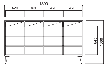
CA-012L W1800・D470・H1010 (W・H1030) (図はアルミ脚)
