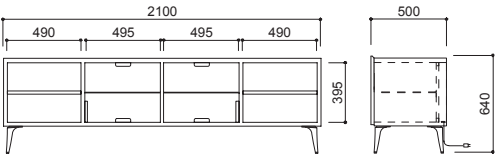
CA-002 Type-B W2100・D500・H640 (W・H660) (図はアルミ脚)
