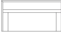
AD-015B-2PL (H720) W1660・D850・SH400
