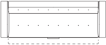
AD-235S(ソファベッド) W2270・D840(980)・H750(SH400)・AH700
