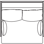
AD-085B-1P W960・D930・H750・SH400
