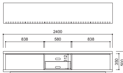
MD-301N-240 W2400×D450×H500
