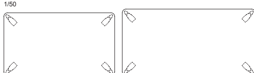
AD-115A(150) W1500-D850-H700(t40)
