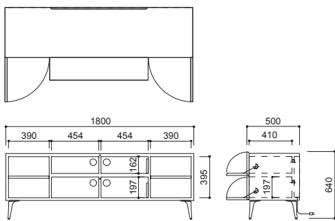
CA-001 Type-A W1800・D500・H640 (W・H660) (図はアルミ脚)
