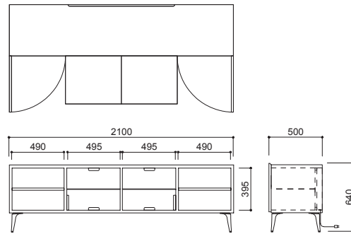
CA-002 Type-B W2100・D500・H640 (W・H660) (図はアルミ脚)
