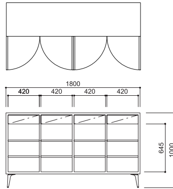
CA-012L W1800・D470・H1010 (W・H1030) (図はアルミ脚)
