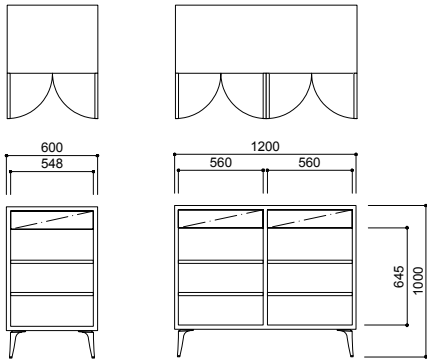
CA-012S W600・D470・ H1010 (W・H1030) (図はアルミ脚)
