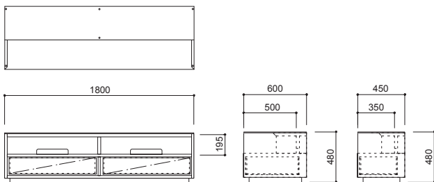
CA-017-HO W1800・D600、450・H480
