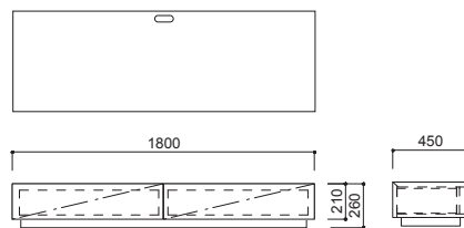
CA-017-L W1800・D600、450・H260
