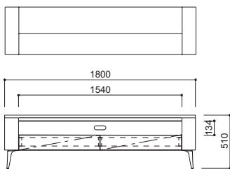
CA-016W-HC W1800・D450・H510 (W・H530) (図はアルミ脚)
