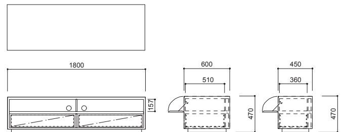
CA-017-HM W1800・D600、450・H470
