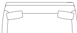
NC-045BC/C-3P W2100 × D875 × H850 (SH400) AH590 (Lクッション×2)
