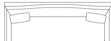
NC-046BC/C-3PL W2400 × D900 × H850 (SH400) AH650 (Lクッション×2)
