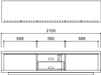
MD-301N-210 W2100・D450・H500
