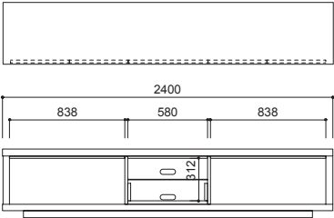
MD-301N-240 W2400・D450・H500
